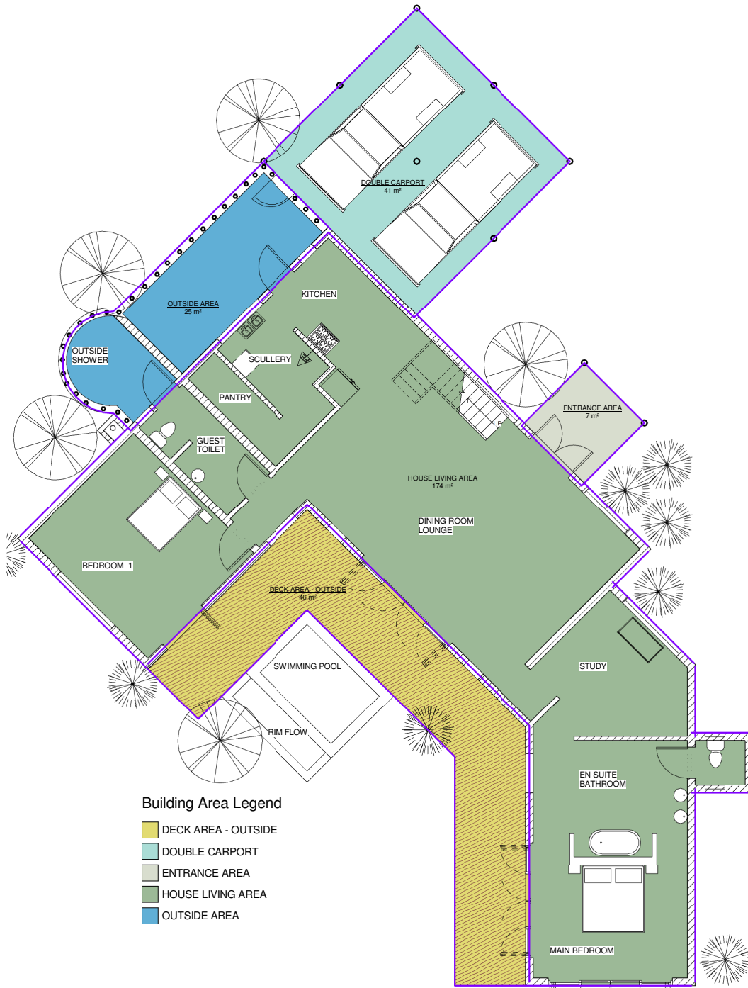
1 AREA PLAN 1 : 50
